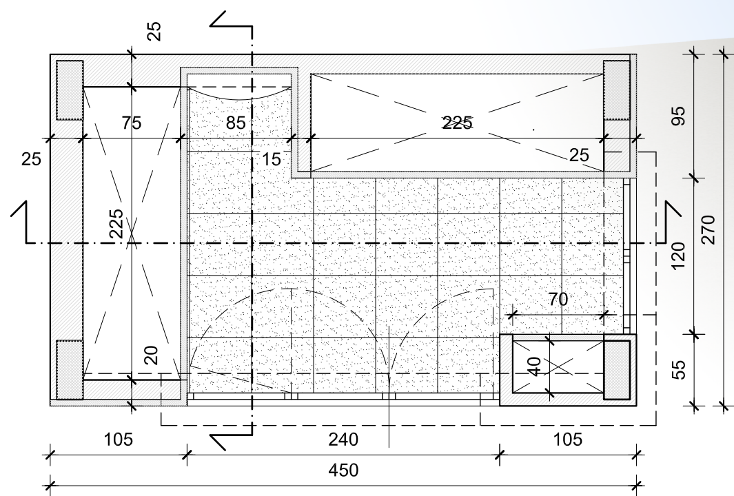
Pianta
