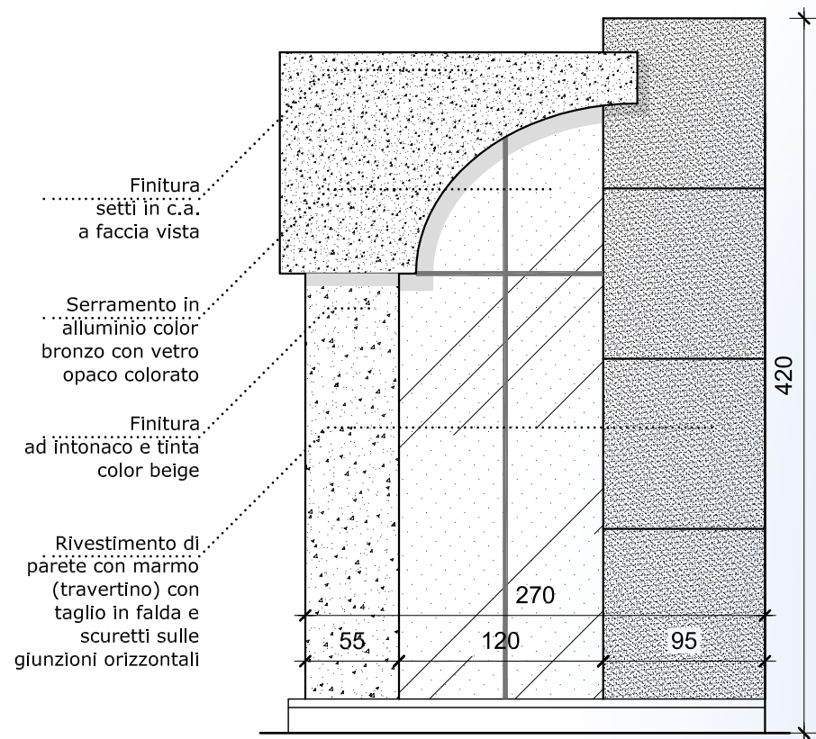
Prospetto
