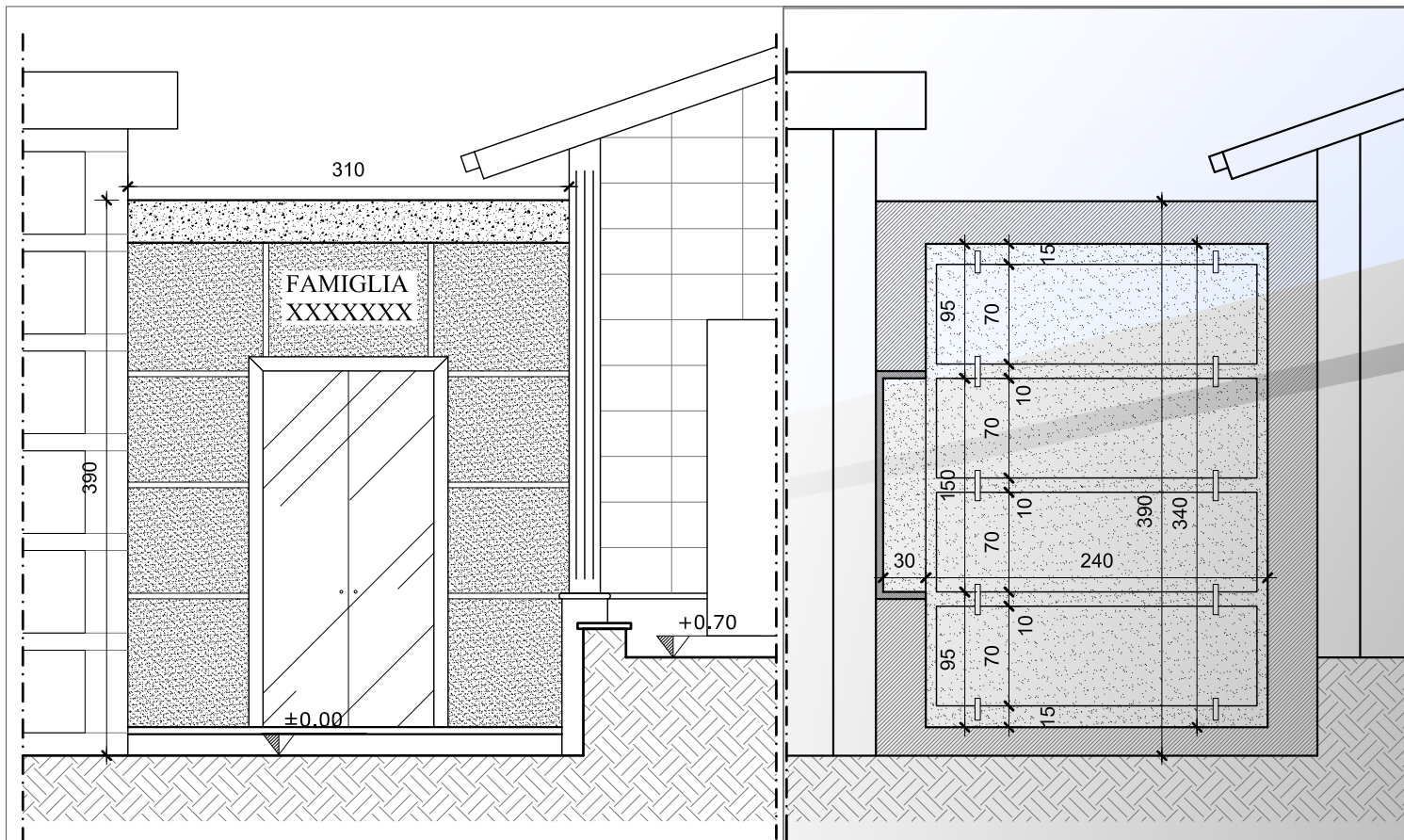
Sezione trasversale
