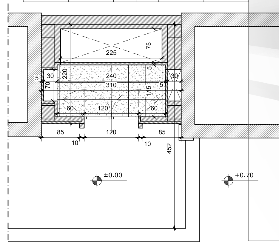
Pianta
